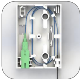
Drop → Fusão → Pigtail → Adaptador
