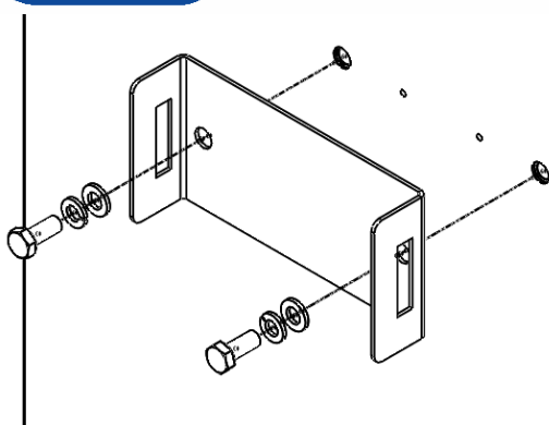
Detalhe 1
