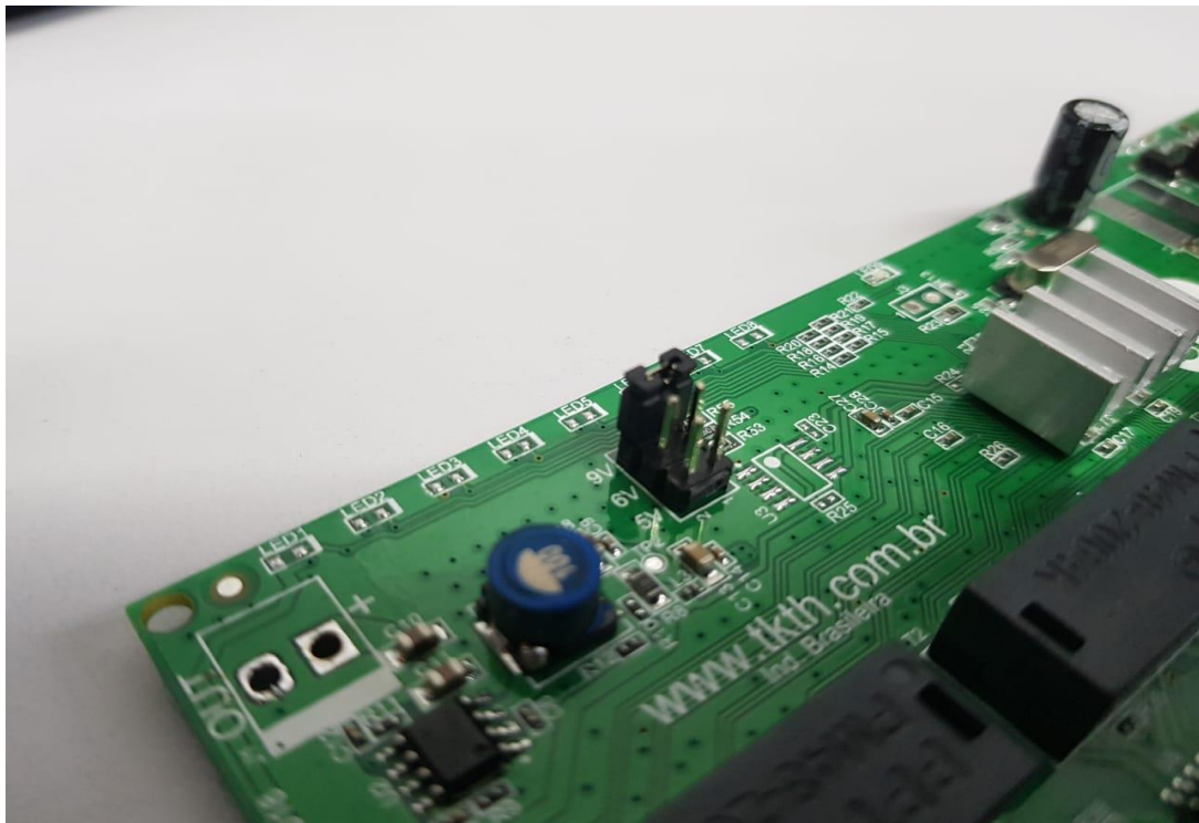
Figura 6- Exemplo de configuração de tensão em 9 VDC – Posição acima.
