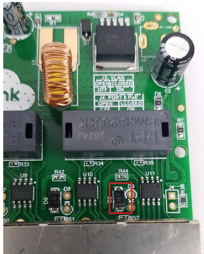
Figura 1-Retirada diodo D2.
