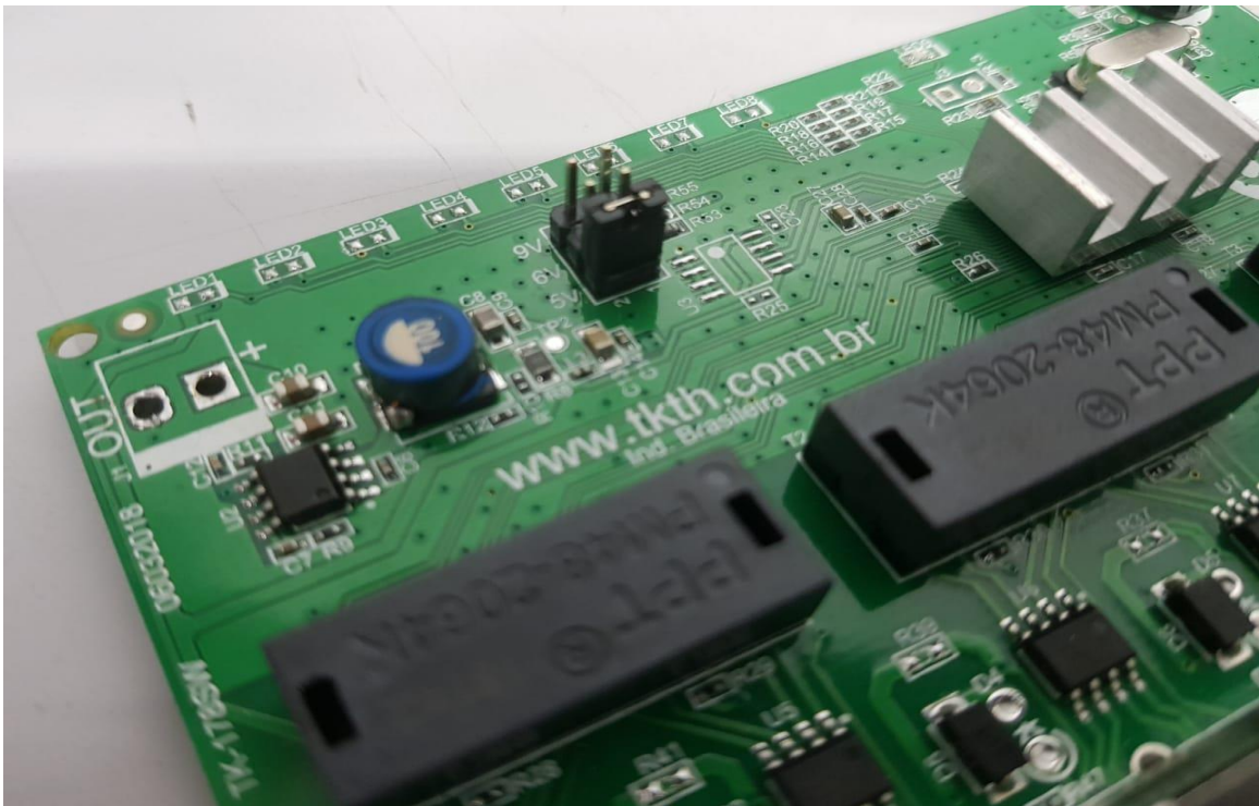
Figura 8-Exemplo de configuração de tensão em 5 VDC – Posição abaixo.
