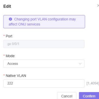
Figura 29: Criação de VLAN
